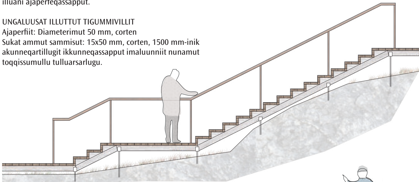
Tummeqqat 27°, 1 : 100, qaffariaataa: 150 mm, toqqavik: 300 mm
