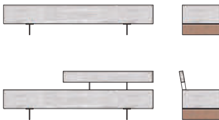
Tunngaviit - Issiaartarfik 1, 1:50, qulaaniit saneraaniillu isigalugu.
