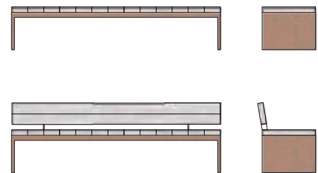
Tunngaviit - Issiaartarfik 2, 1:50, qulaaniit saneraaniillu isigalugu.
